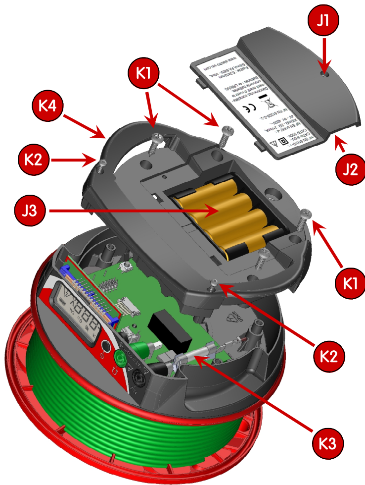
VUE ECLATÉE.
