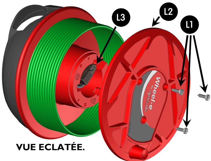
VUE ECLATÉE.
